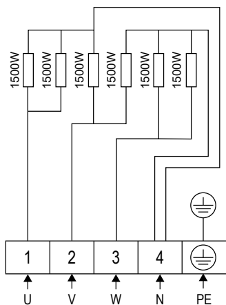
Figura 5. Schema elettrico QU90E
