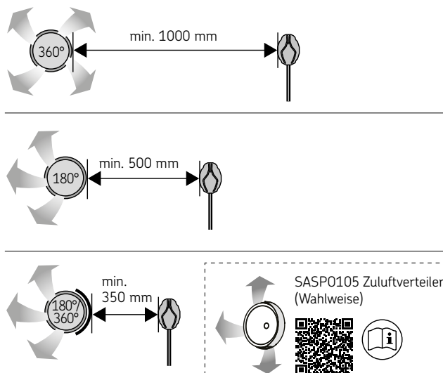
Rysunek 10. Minimalna odległość otworu wentylacyjnego od czujnika.
