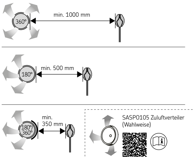
Figuur 10. Minimale afstand van de luchttoevoerklep tot de temperatuursensor.
