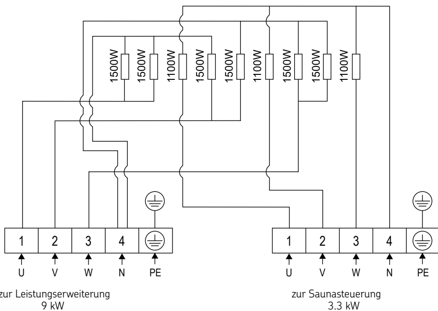
Abbildung 7. Verdrahtungsschema QU120E
