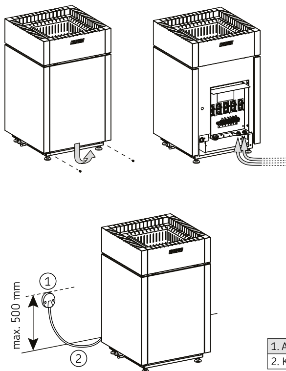
Figuur 4. Elektrische aansluitingen
