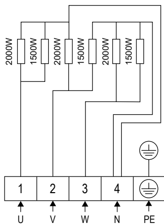
Kuva 6. Kytentäkaavio QU105E
