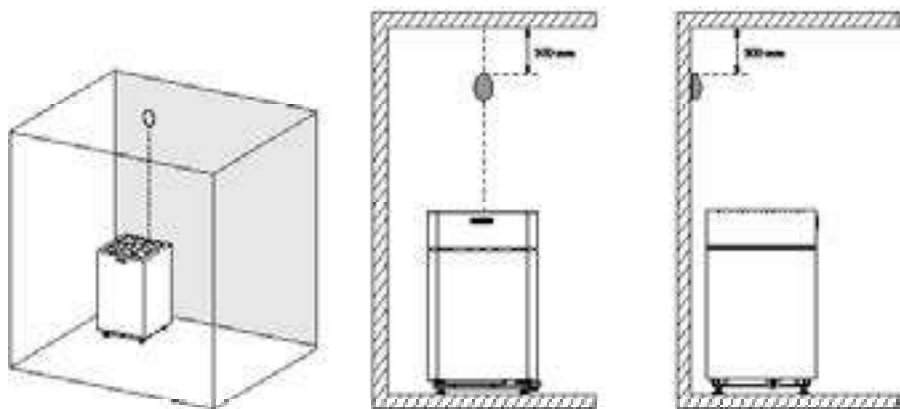
Joonis 3a. Soojusanduri paigaldamine seinal
