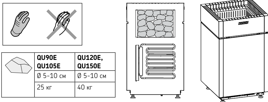
Рисунок 9. Наполнение каменки камнями
