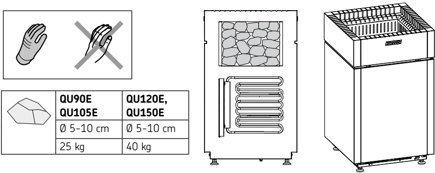
Figura 9. Colocación de las piedras de la sauna
