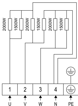
Figuur 6. Aansluitschema QU105E
