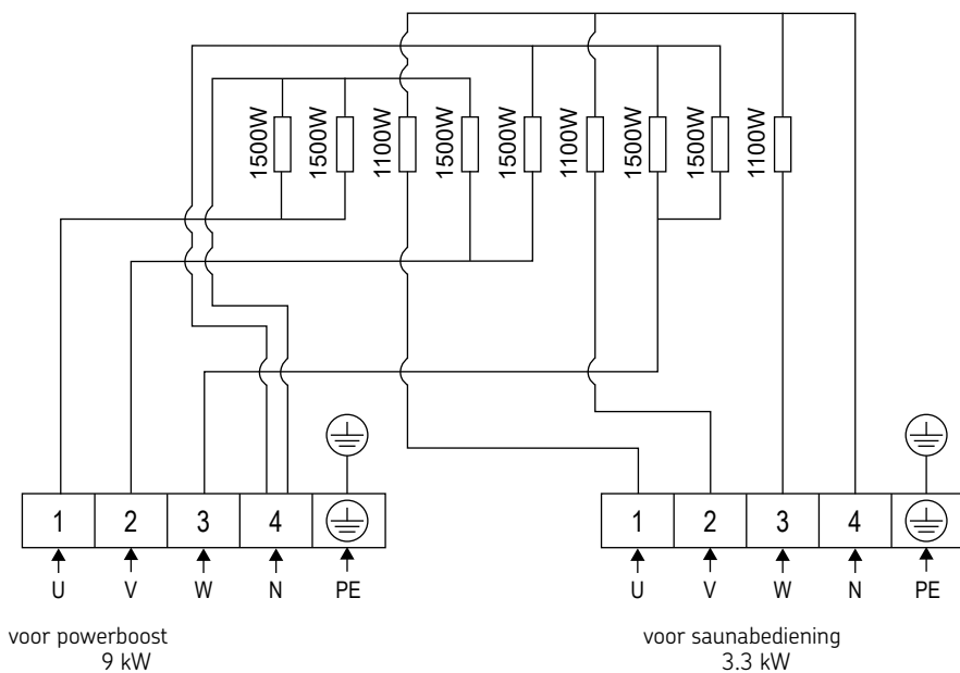
Figuur 7. Aansluitschema QU120E
