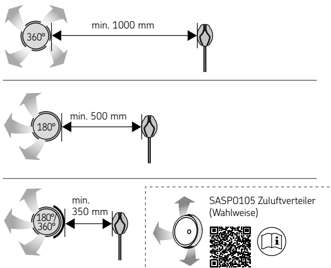
Abbildung 10. Mindestabstand des Fühlers zur Luftzufuhr.
