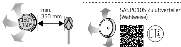
10 pav. Mažiausias atstumas nuo tiekiamo oro ventiliacijos angos iki temperatūros jutiklio
