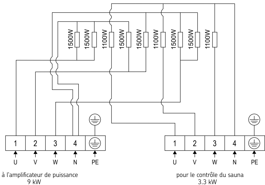
Figure 7. Schéma de câblage QU120E
