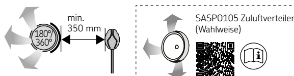
Figura 10. Distanza minima tra lo sfiato dell'aria di alimentazione e il sensore di temperatura.
