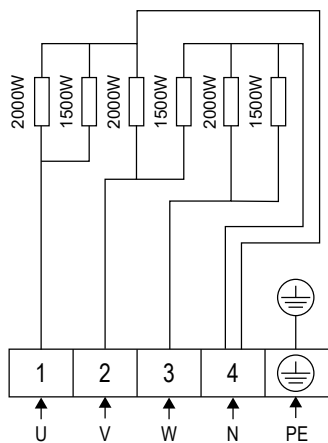
Slika 6. Shema ožičenja QU105E
