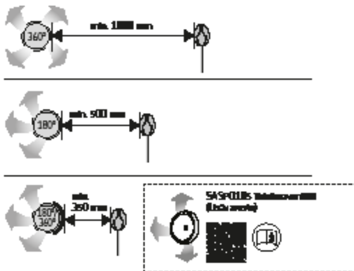
Kuva 10. Tuloilmaventtiilin vähimmäisetäisyys lämpötila-anturiin
