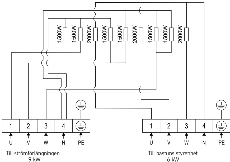
Bild 8. Kopplingsschema QU150E
