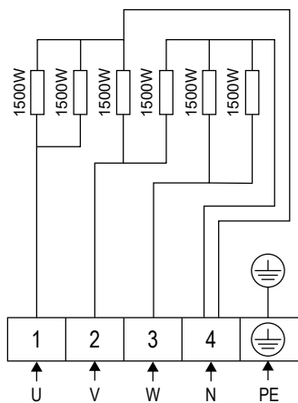
5. attēls. Elektroinstalācijas shēma QU90E
