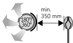
Obrázek 10 Minimální vzdálenost od větracího otvoru přívodu vzduchu k teplotnímu senzor
