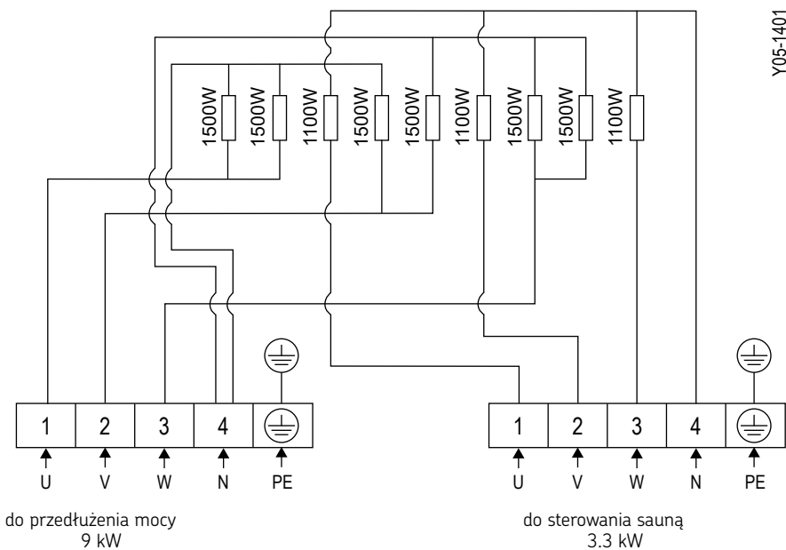
Rysunek 7. Schemat połączeń QU120E
