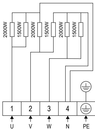
6 pav. Laidų prijungimo schema QU105E
