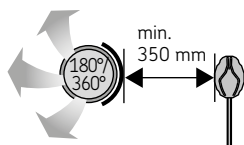
Рисунок 10. Минимальное расстояние от температурного датчика до вентиляционной отдушины.
